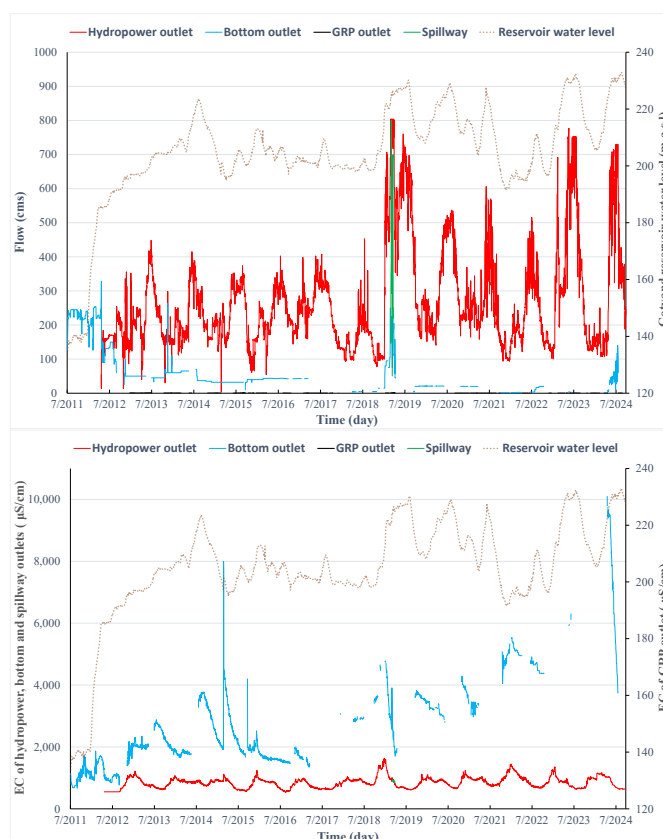
شکل ۱۲- مقادیر جریان خروجی (الف) و شوری جریان خروجی (ب) از مخزن سد گتوند به تفکیک سازه‌های مختلف در طول دوره بهره‌برداری Figure 12- Outflow discharge (a) and outflow salinity (b) from Gotvand Dam reservoir, according to individual outlet structures throughout the operation period.
