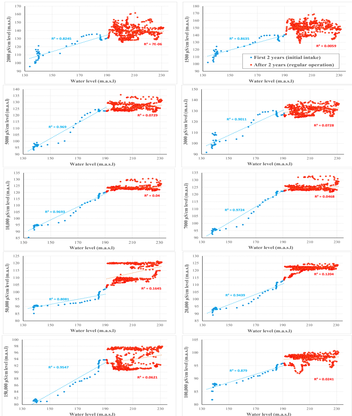
شکل ۴- ارتباط بین تراز آب مخزن با تراز قرارگیری لایه‌های با شوری مختلف ( \mu\text{S/cm} ) به تفکیک دوره آبگیری و دوره بهره‌برداری مخزن سد گتوند
