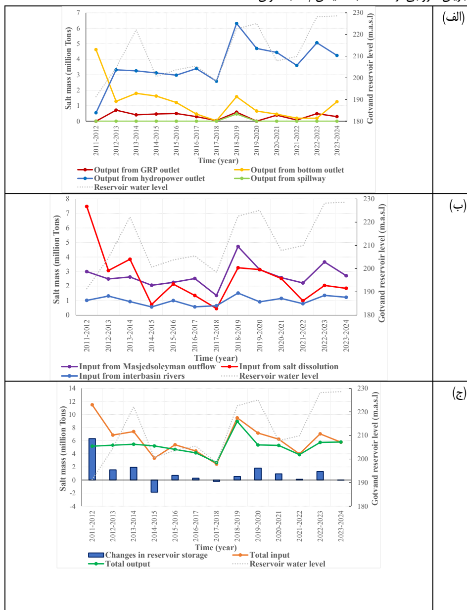
شکل ۱۳- (الف) جرم سالانه نمک خروجی مخزن سد گتوند به تفکیک دریاچه‌های مختلف، (ب) جرم سالانه نمک ورودی به مخزن سد گتوند به تفکیک منبع، و (ج) وضعیت سالانه مؤلفه‌های اصلی بیلان نمک در مخزن سد گتوند.
