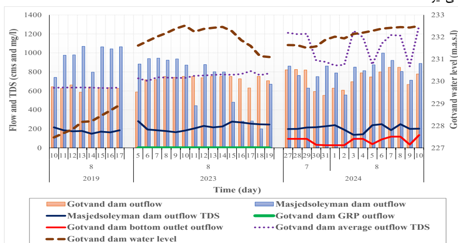
شکل ۶- مقادیر متوسط روزانه جریان خروجی از سد های گتوند و مسجدهسلیمان در ۳ بازه زمانی دارای جریان‌های ورودی نسبتاً بالا از مخزن سد
