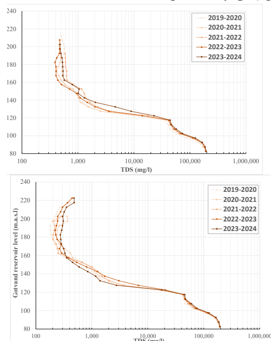
شکل ۱۰- تغییرات شوری در عمق مخزن سد گتوند در دوره ۵ ساله ۱۳۹۹-۱۴۰۳ برای (الف) انتهای فصل سرد و (ب) انتهای فصل گرم Figure 10- Salinity variations along the depth of the Gotvand Dam reservoir over the five-year period 2020-2024, for (a) the end of the cold season and (b) the end of the warm season.
