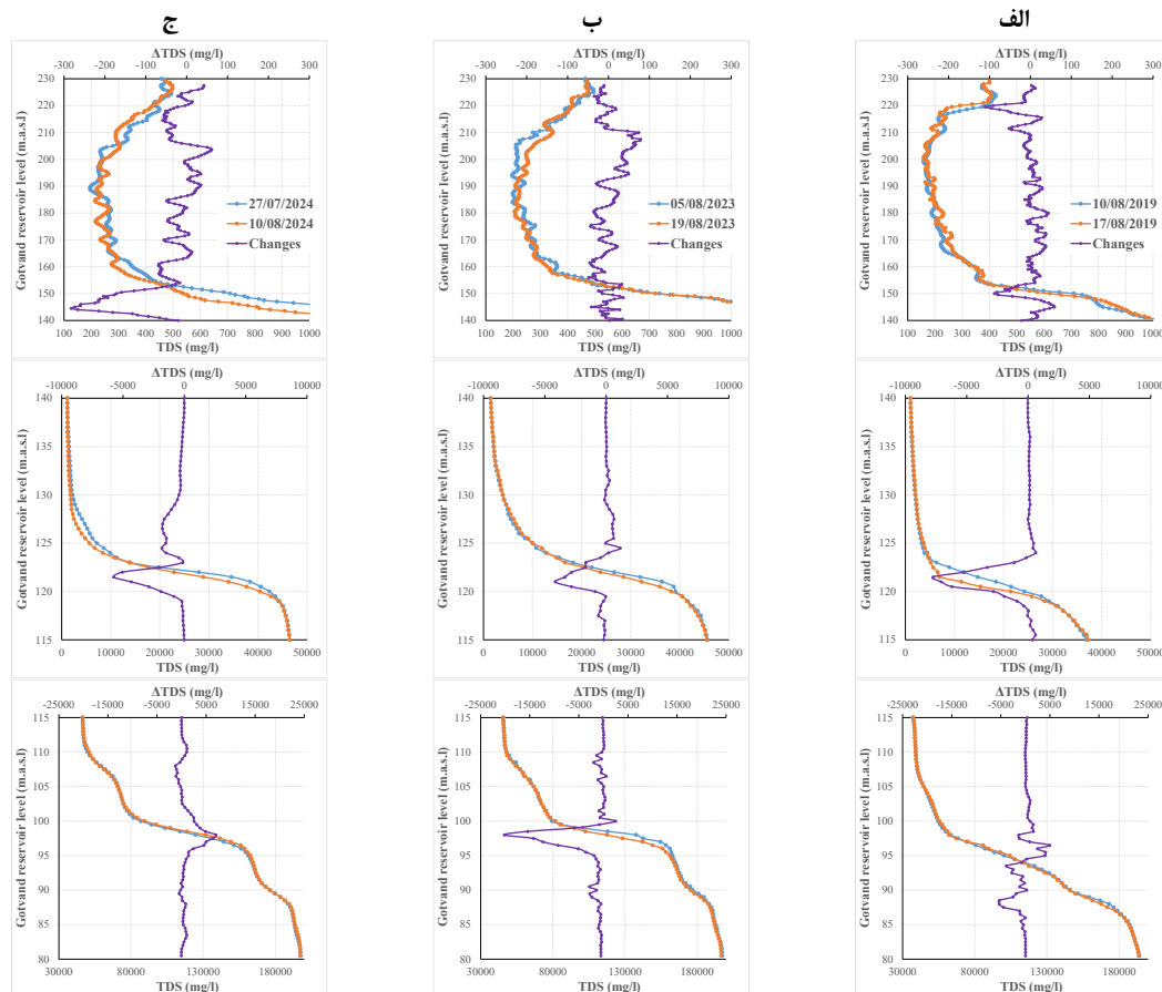
شکل ۷- وضعیت شوری در عمق مخزن سد گتوند به تفکیک سه بازه عمقی مختلف (ردیف‌های ۱ تا ۳) در ابتدا و انتهای بازه‌های زمانی مورد ارائه در شکل ۶ (ستون‌های الف و ب و ج)
