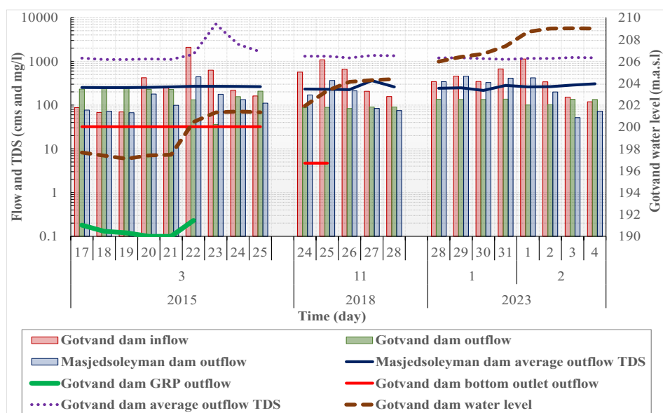
شکل ۸- مقادیر متوسط روزانه جریان خروجی از سد‌های گتوند و مسجدسلیمان در سه رخداد سیلابی میان‌حوضه، وضعیت تخلیه جریان از GRP و تخلیه‌کننده تحتانی، شوری جریان ورودی به مخزن گتوند و تغییرات تراز آب آن
