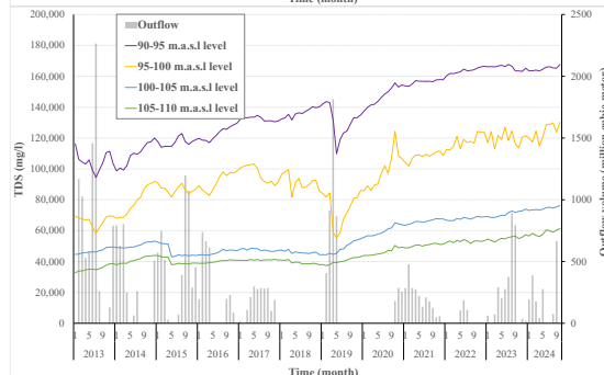
شکل ۱۱- مقادیر ماهانه جریان خروجی از آبیگر نیروگاه (الف)، آبیگر تحتانی (ب) و GRP (ج) و اثر آنها بر TDS متوسط لایه‌های نزدیک به
