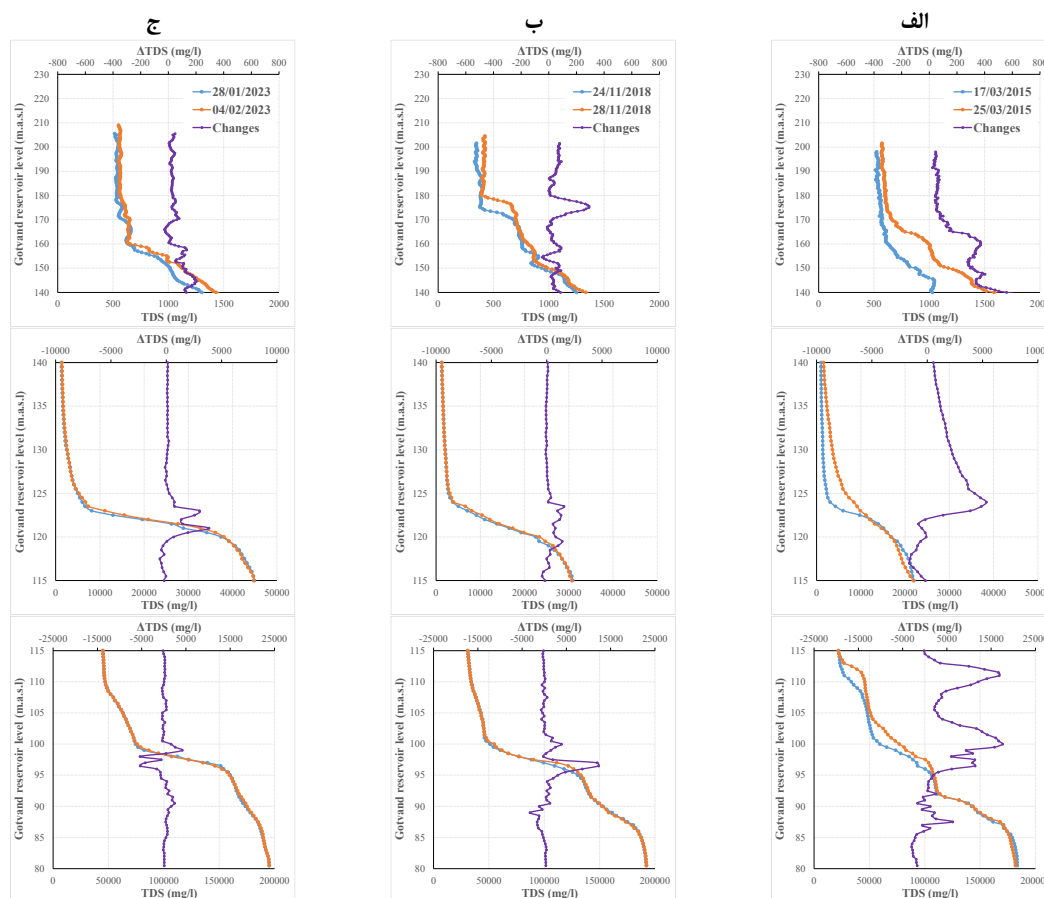
شکل ۹- وضعیت شوری در عمق مخزن سد گتوند به تفکیک ۳ بازه عمقی مختلف (ردیف‌های ۱ تا ۳) در ابتدا و انتهای بازه‌های زمانی مورد ارائه در شکل ۸ (ستون‌های الف و ب و ج)
