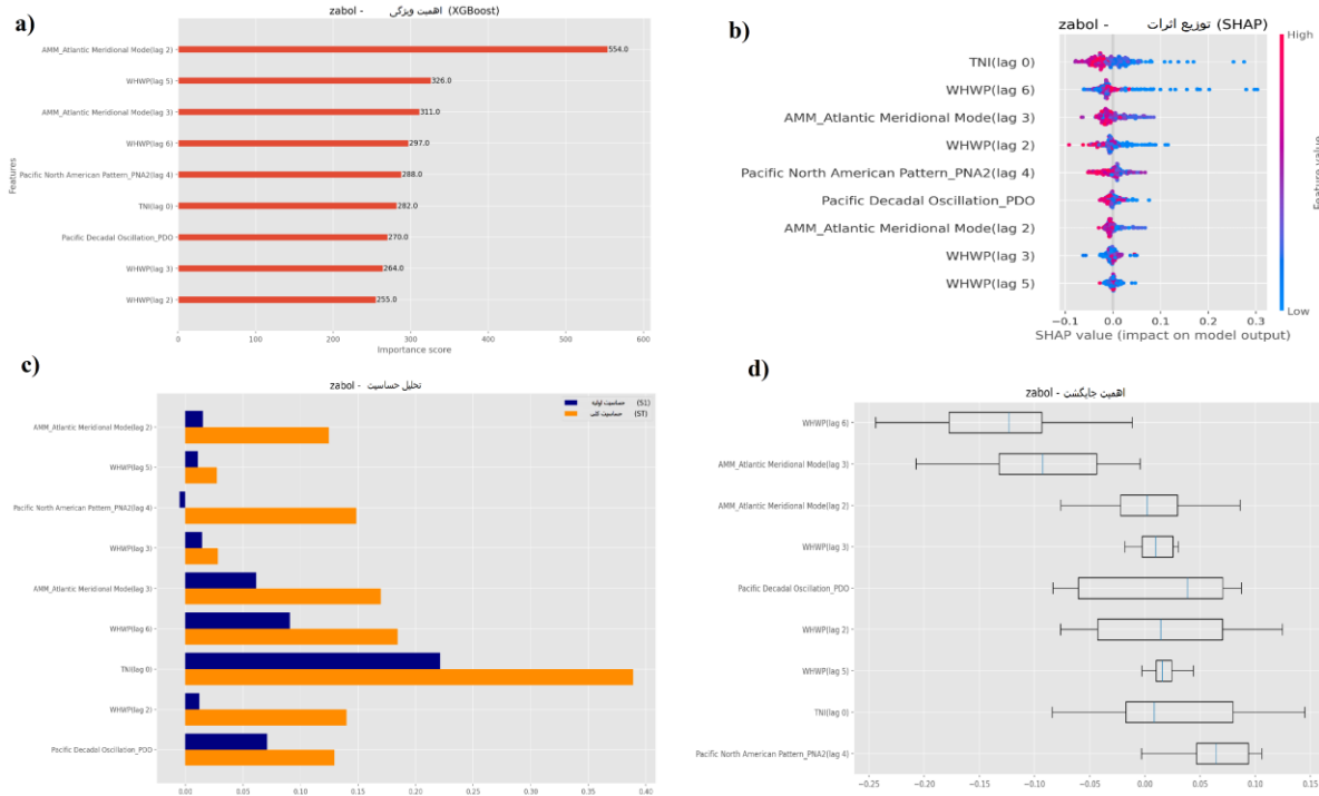
شکل ۹- الف) نمودار اهمیت ویژگی ب) تغییرات شاخص‌های اقلیمی با روش SHAP پ) تحلیل حساسیت شاخص‌ها با روش Sobol ت) تحلیل اهمیت جایگزینی شاخص‌ها در ایستگاه زابل
