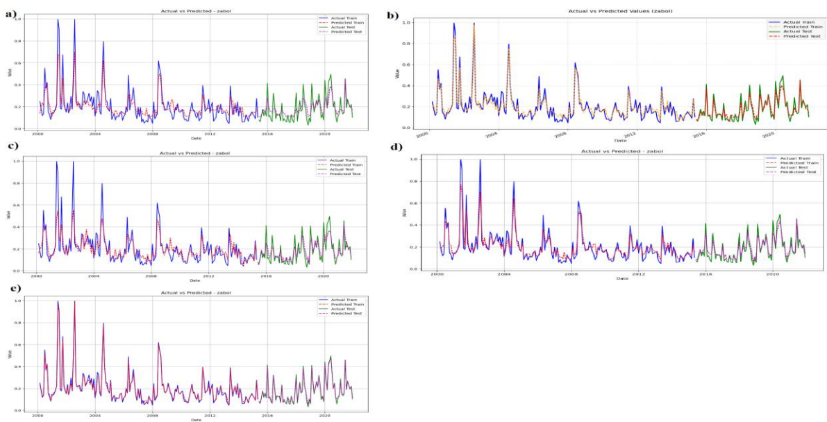
شکل ۶- پیش‌بینی AOD با مدل‌های الف) Bagged CART ب) Gradient Boosting پ) LightGBM ت) Random Forest ث) XGBoost در ایستگاه زابل
