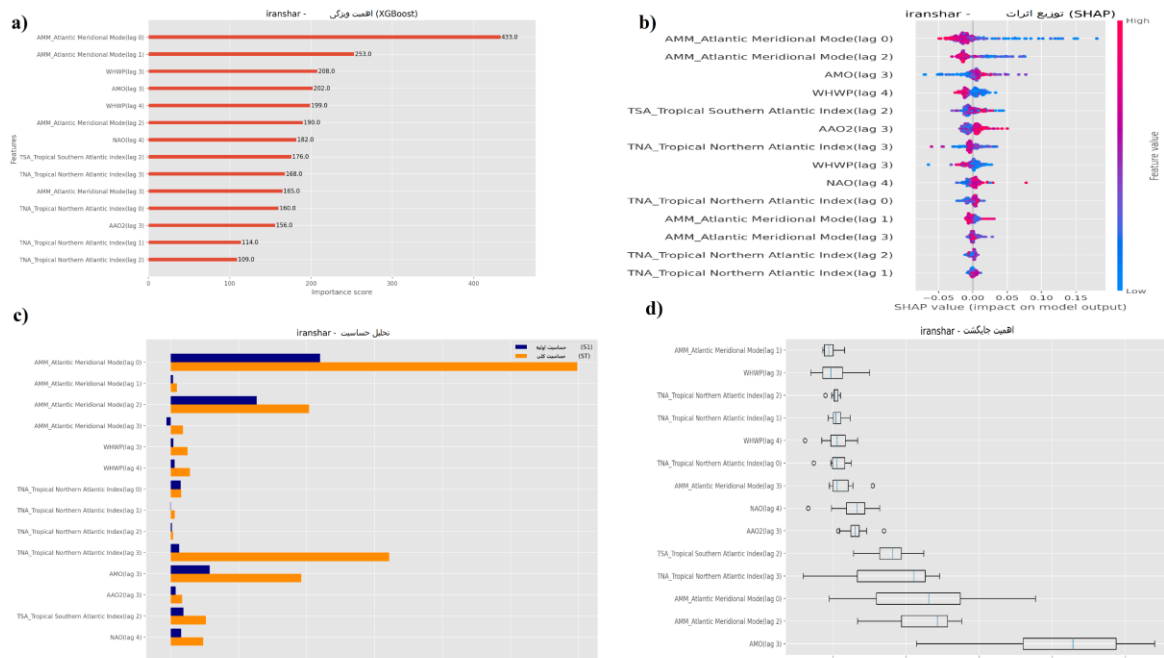
شکل 7- الف) نمودار اهمیت ویژگی ب) تغییرات شاخص‌های اقلیمی با روش SHAP پ) تحلیل حساسیت شاخص‌ها با روش Sobol ت) تحلیل اهمیت جایگشت شاخص‌ها در ایستگاه ایرانشهر
