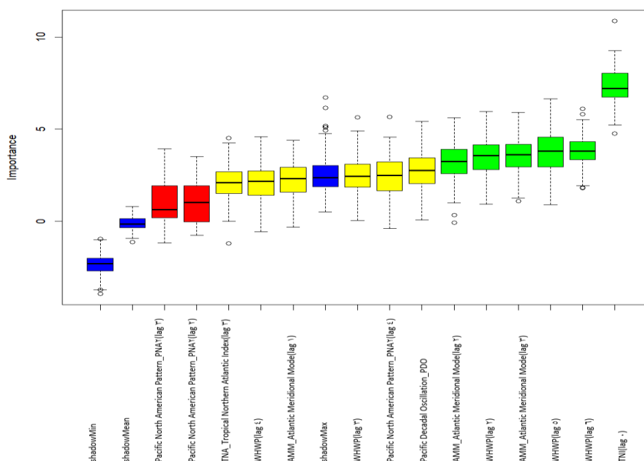
شکل 4- شاخص‌های پیوند از دور مؤثر بر AOD در ایستگاه زابل با استفاده از الگوریتم Boruta Figure 4- Effective teleconnection indices on AOD at Zabol station using the Boruta algorithm
