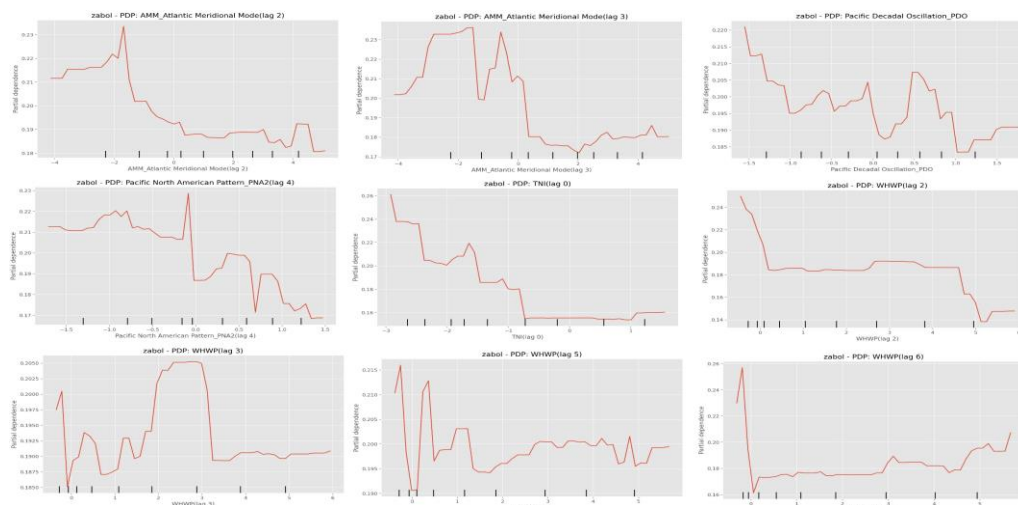
شکل 10- بررسی رفتار مدل در برابر تغییرات شاخص های اقلیمی با استفاده از تحلیل PDP در ایستگاه زابل Figure 10- Investigating the behavior of the model against changes in climatic indicators using PDP analysis at Zabol station
