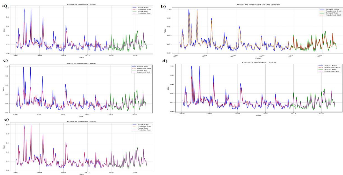
شکل 6- پیش‌بینی AOD با مدل‌های الف) Bagged CART ب) Gradient Boosting پ) LightGBM ت) Random Forest ث) XGBoost در ایستگاه زابل
