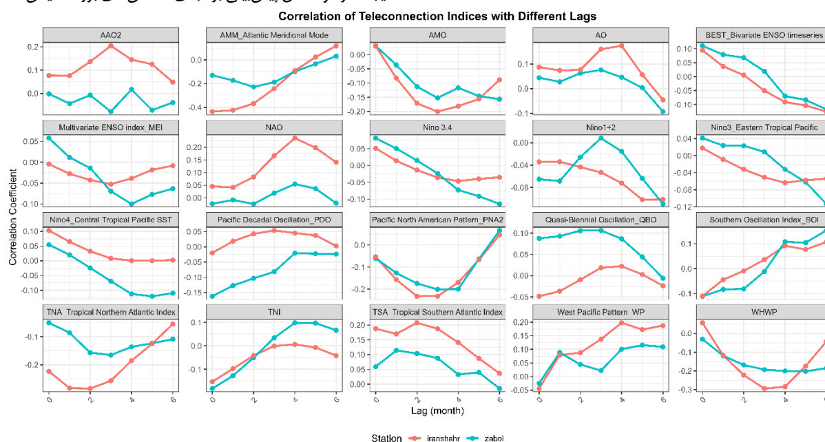
شکل 2- همبستگی شاخص های پیوند از دور در تأخیرهای مختلف با AOD در ایستگاه های ایران شهر و زابل Figure 2- Correlation of teleconnections indices at different lags with AOD at Iranshahr and Zabol stations
