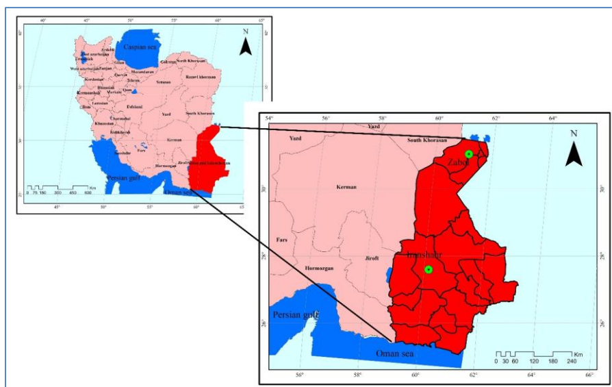
شکل 1- منطقه مورد مطالعه
