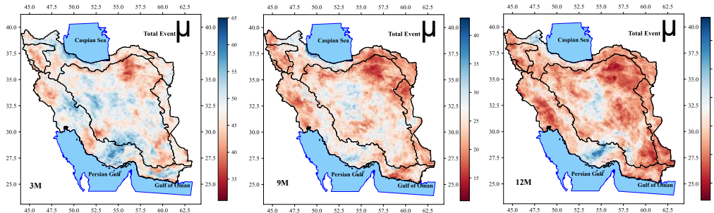
۵- توزیع مکانی تعداد رخدادهای خشکسالی بر اساس شاخص SPEI در مقیاس‌های ۳، ۹ و ۱۲ ماهه Figure 5. Spatial distribution of SPEI-based drought events at 3-, 9-, and 12-month scales
