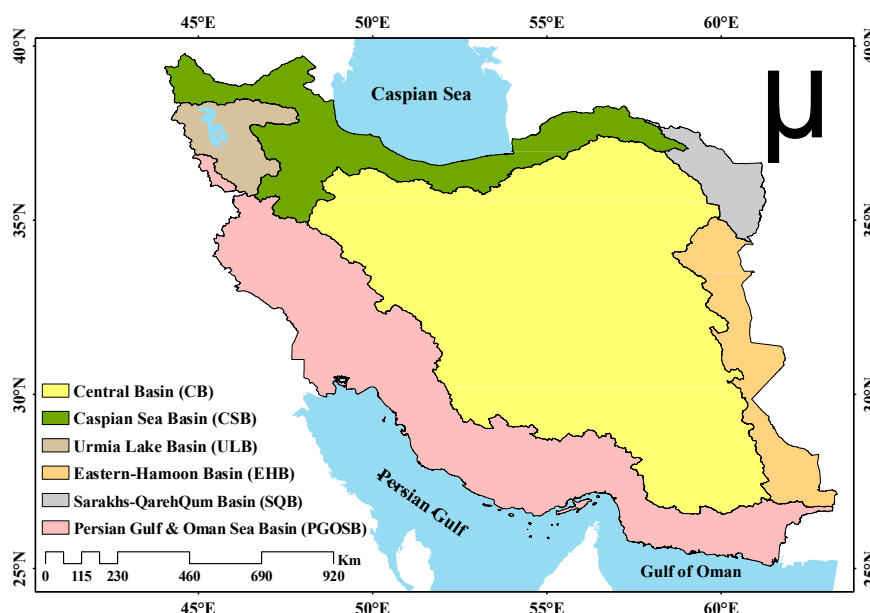
شکل ۱- موقعیت جغرافیایی و مرزهای شش حوضه آبریز اصلی ایران Figure 1. Geographical location and boundaries of the six major basins in Iran
