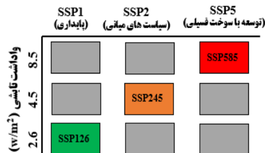
شکل ۲- سناریوهای SSP و میزان واداشت تابشی (O'Neill et al. 2017)
