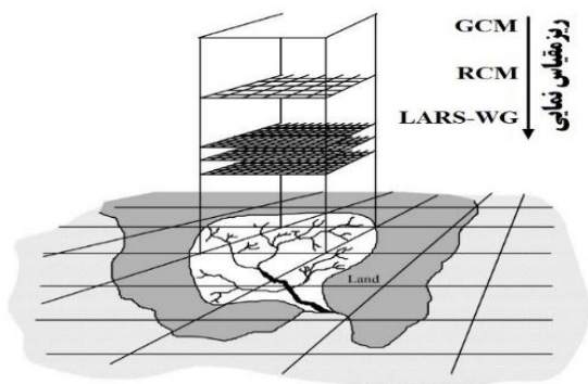
شکل ۳- ریزمقیاس نمایی مدل‌های گردش عمومی Figure 3- Downscaling general circulation models
