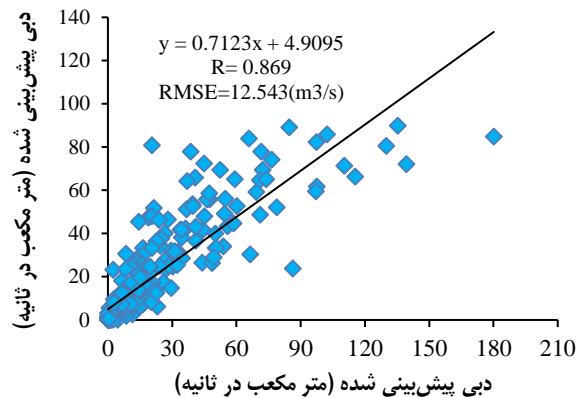
شکل ۶- نمودارهای مقادیر مشاهداتی و پیش‌بینی شده حاصل از بهترین مدل SVM در مرحله آموزش
