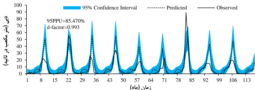
شکل ۹- مقادیر مشاهداتی و پیش‌بینی شده حاصل از مدل ANN و باند اطمینان ۹۵ درصد در مرحله صحت‌سنجی
