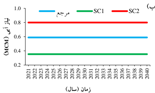
شکل ۸- میزان تقاضای نقطه نیاز شهر تبریز (الف) و کشاورزی نهند (ب) برای دوره ۲۰۲۱-۲۰۴۰ تحت سناریوهای تدوین شده در مدل WEAP در حوضه آبریز نهند
