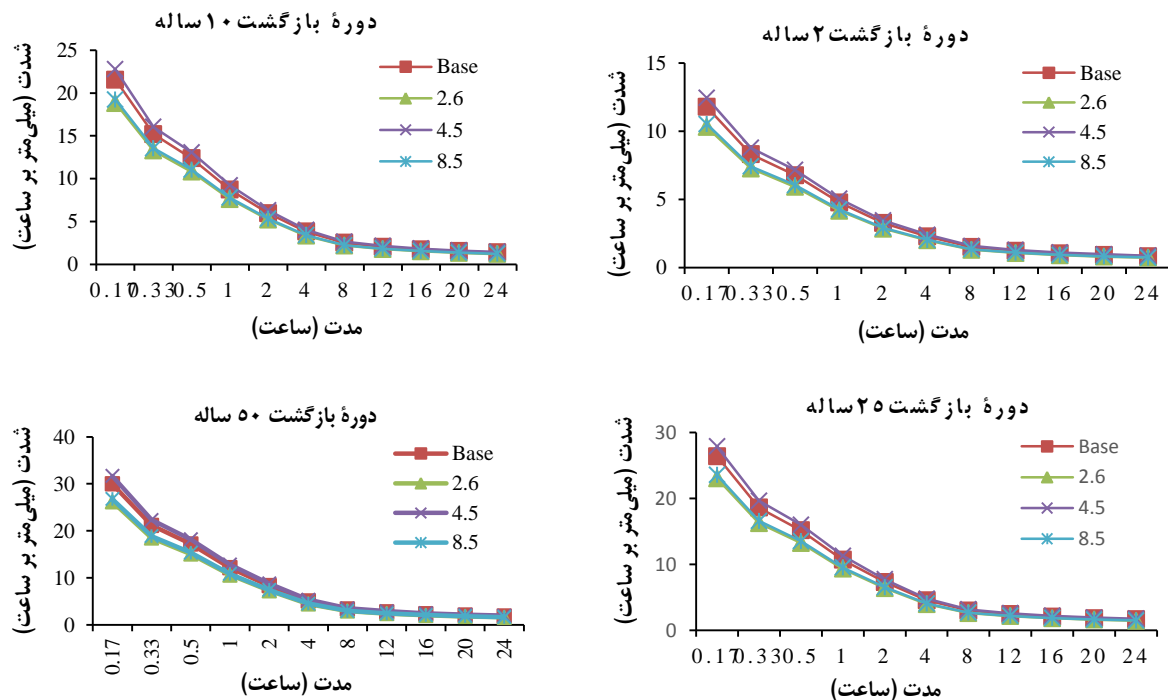
شکل ۹- مقایسه شدت بارندگی در دوره بازگشت های دو، ۱۰، ۲۵، ۵۰ ساله دوره مشاهداتی (۱۹۹۳-۲۰۱۷) با دوره آینده دور (۲۰۵۱-۲۰۷۰) (۲۰۷۰-۲۰۵۱)
