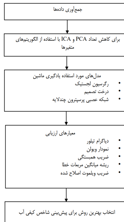
شکل ۲- نمودار مراحل انجام مدل‌سازی شاخص WQI
