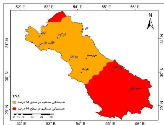
شکل ۱۴- همبستگی متوسط دمای حوضه و الگوی TNA در مارس Figure 14- Correlation of average basin temperature and TNA pattern in March
