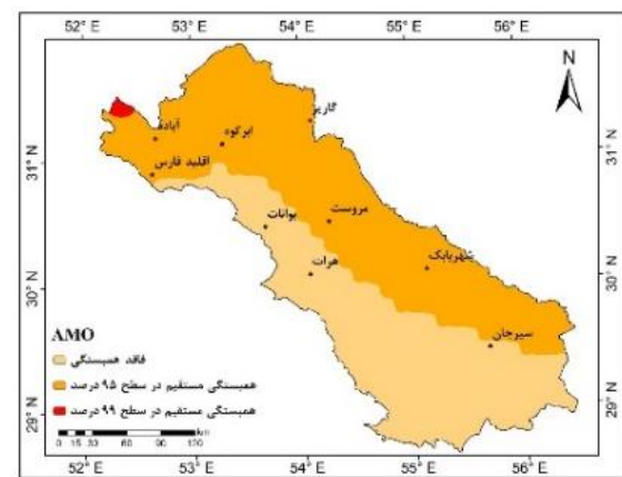
شکل ۲۰- همبستگی متوسط دمای حوضه و الگوی AMO در آوریل Figure 20- Correlation of average basin temperature and AMO pattern in April
