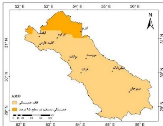
شکل ۲۳- همبستگی متوسط دمای حوضه و الگوی AMO در ژوئن Figure 23- Correlation of average basin temperature and AMO pattern in June
