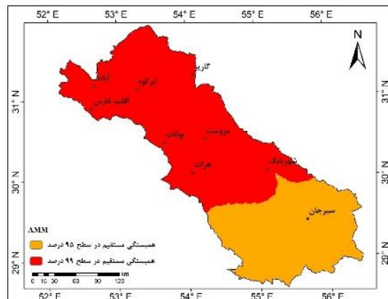
شکل ۲۸- همبستگی متوسط دمای حوضه و الگوی AMM در سپتامبر Figure 28- Correlation of average basin temperature and AMM pattern in September
