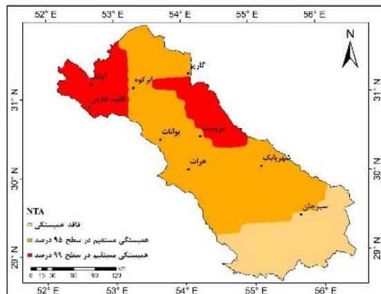
شکل ۱۳- همبستگی متوسط دمای حوضه و الگوی NTA در فوریه Figure 13- Correlation of average watershed temperature and NTA pattern in February
