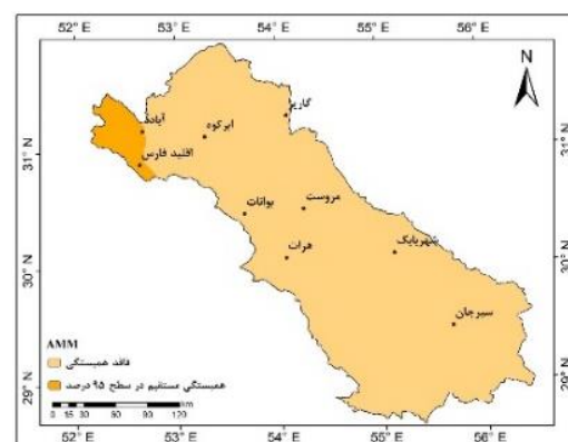
شکل ۳۰- همبستگی متوسط دمای حوضه و الگوی AMM در نوامبر Figure 30- Correlation of average basin temperature and AMM pattern in November
