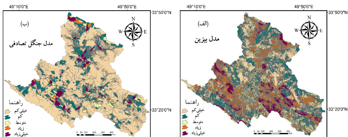
شکل ۴- مناطق مستعد تغذیه آب‌های زیرزمینی طبقه‌بندی شده، (الف) تئوری بیزین و (ب) مدل جنگل تصادفی Figure 4- Groundwater recharge potential zones, (a) Bayesian Theory, and (b) Random forest models (reclassified in ArcGIS 10.6)
