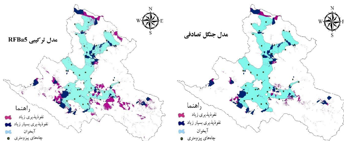
شکل ۷- برازش وضعیت نفوذپذیری با موقعیت آبخوان و چاه‌های پیرومتری حوزه Figure 7 – Overlaying the Marboreh GWR potential map with aquifer layer and pisometric wells
