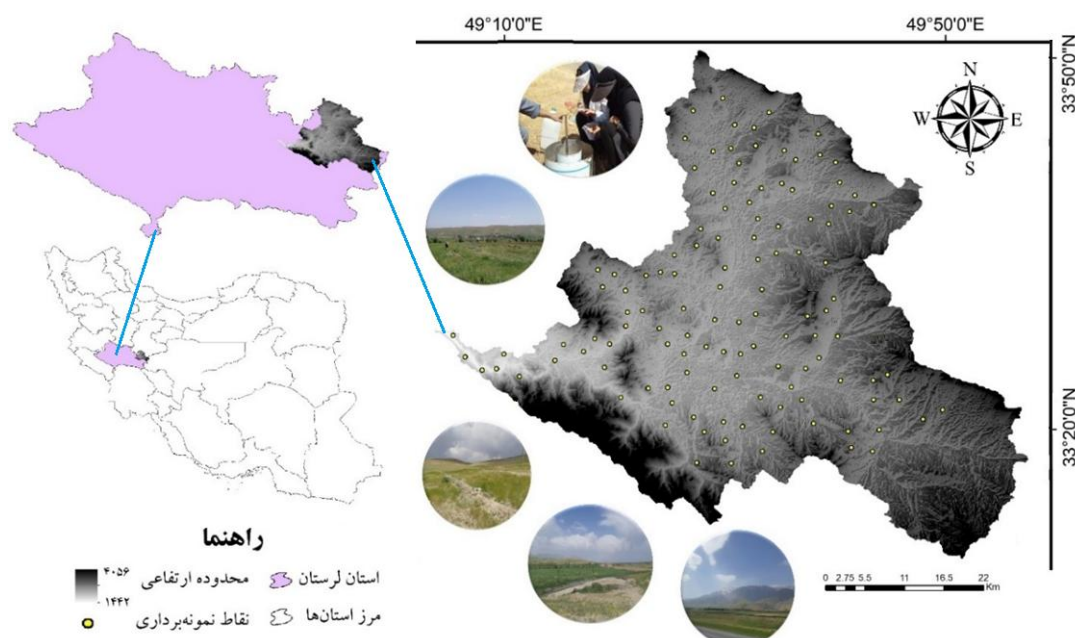
شکل ۱- موقعیت حوزه آبخیز ماربره و نقاط نمونه‌برداری، استان لرستان، ایران Figure 1- Location of Marboreh Watershed and field survey samples, Lorestan Province, Iran
