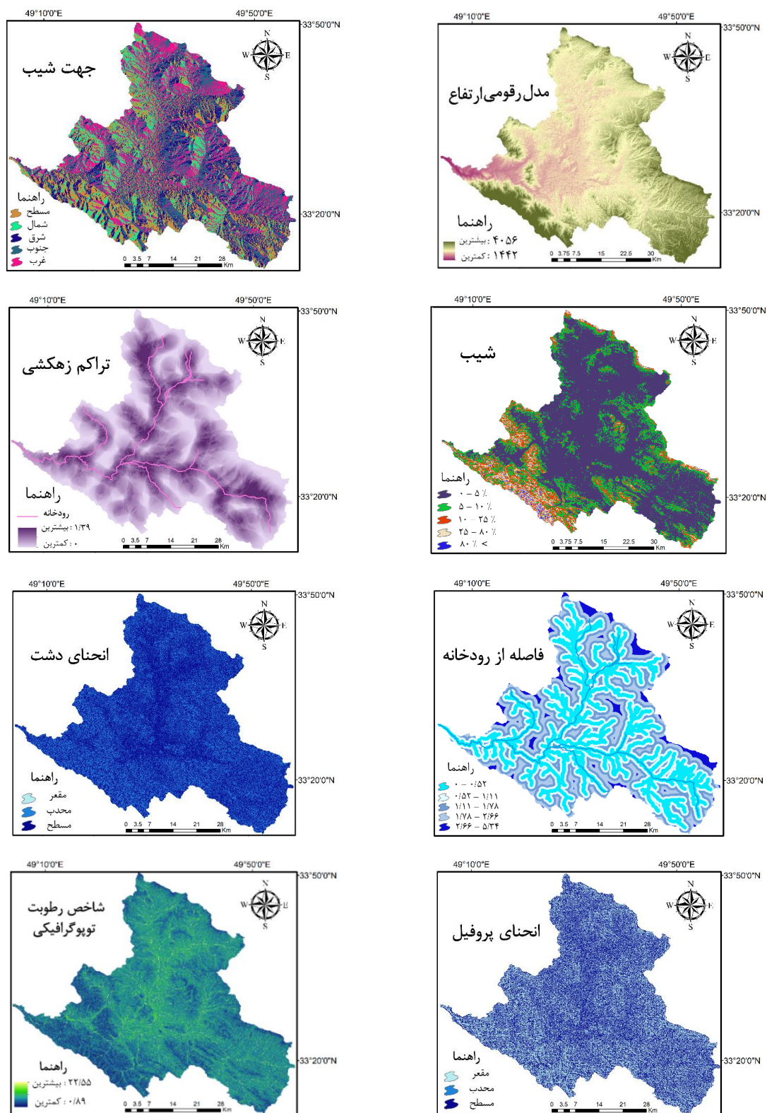
شکل ۲- لایه های اطلاعات محیطی حوزه آبخیز ماربره
