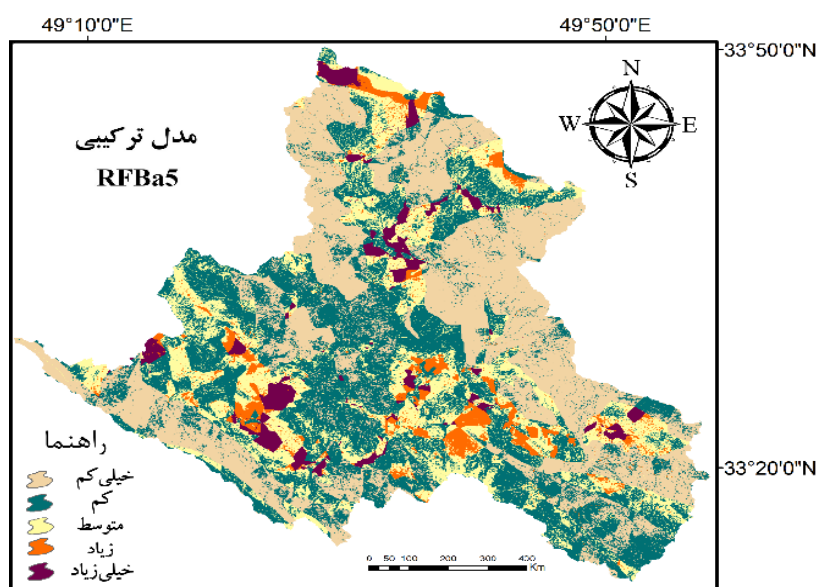
شکل ۵- مناطق مستعد تغذیه آب‌های زیرزمینی طبقه‌بندی شده طبق مدل ترکیبی RFBa5 Figure 5 – Groundwater recharge potential zones according to RFBa5 ensembling scenario
